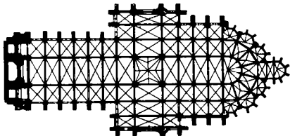
99. Собор в Амьене. План
